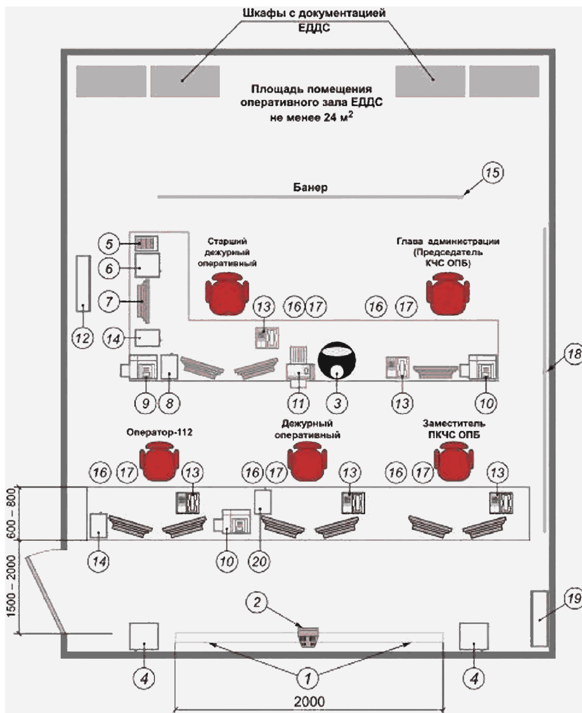
Рисунок А.1 - Примерная схема размещения рабочих мест и оборудования ЕДДС
