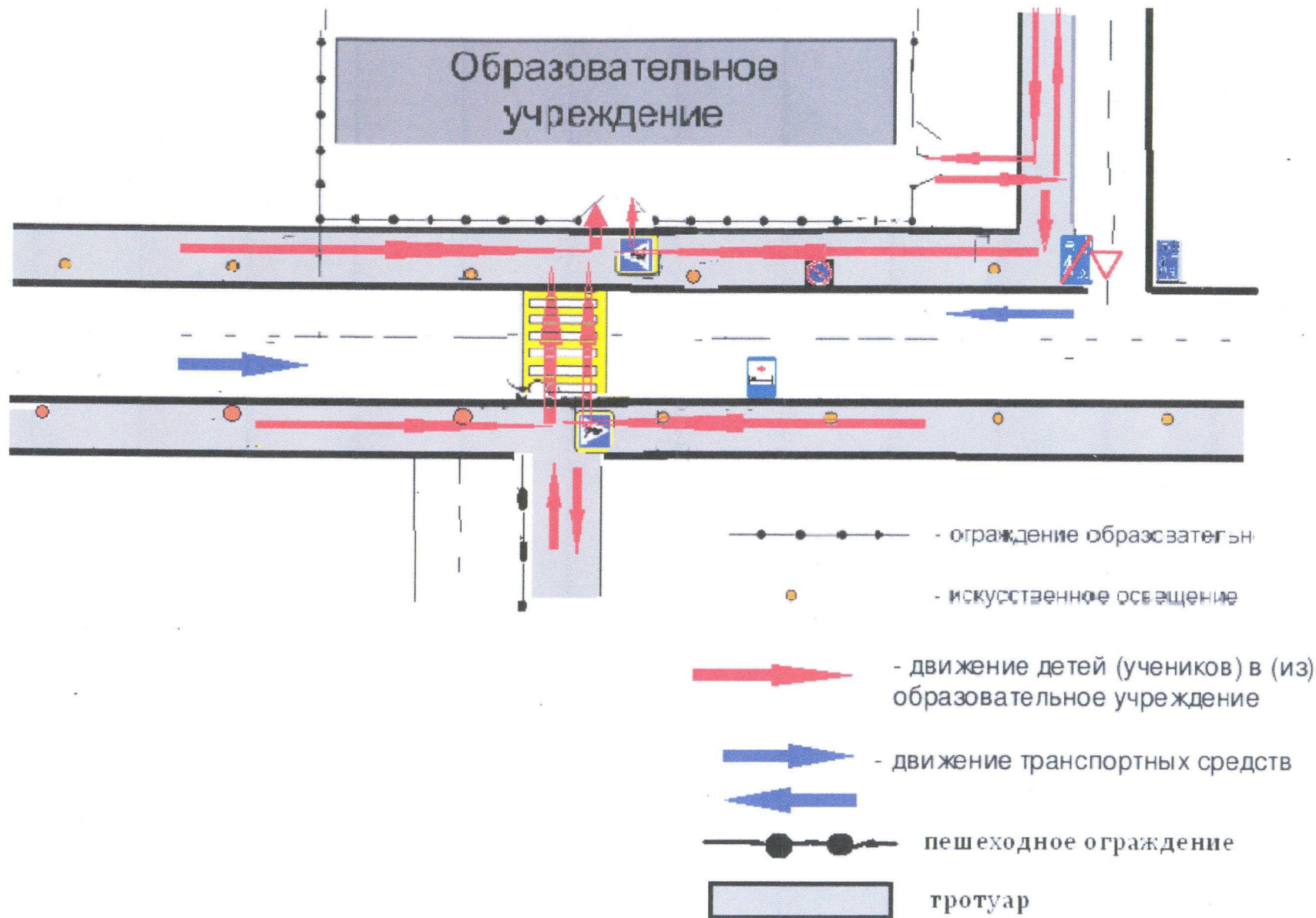
Схема организации дорожного движения на нерегулируемом пешеходном переходе в непосредственной близости от образовательного учреждения при двухполосном движении транспортных средств.
