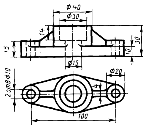
Фланец
