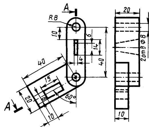
Замок
