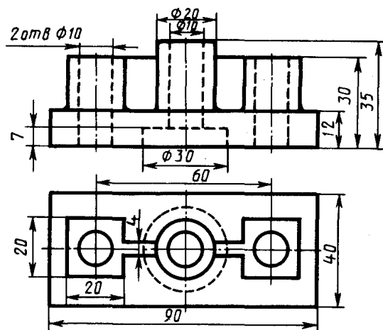
Опора
