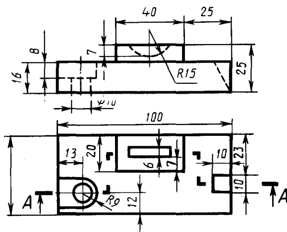
Брусок
