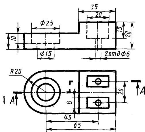
Упор
