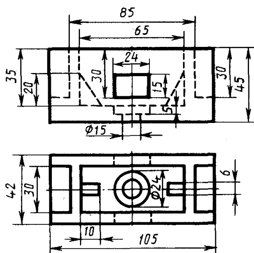
Коробка
