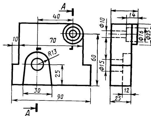
Стойка
