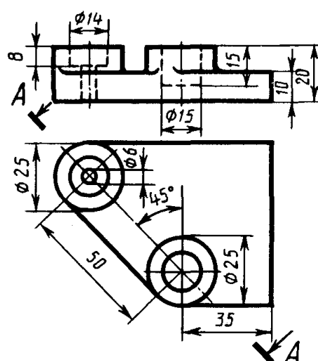
Плита
