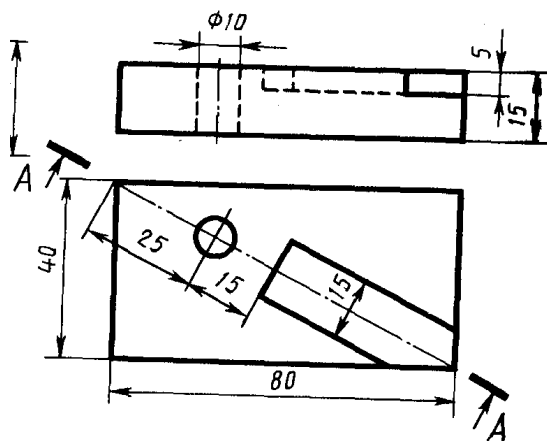
Плита
