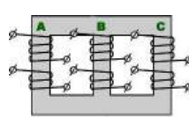
схема построения трехфазного трансформатора Трансформатор Суханова
