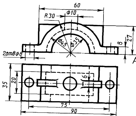
Крышка
