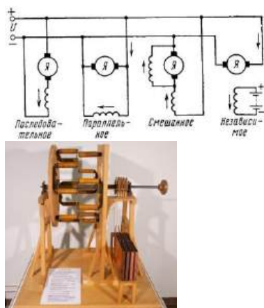
ДВИГАТЕЛЬ ПОСТОЯННОГО ТОКА
