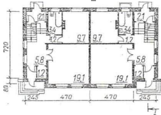
П ген 1-го этажа
