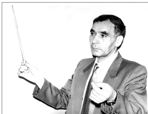
И.Егоров
