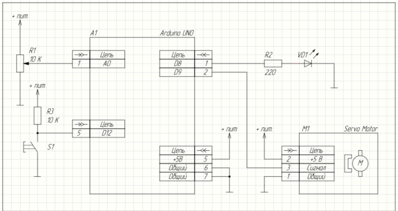
Рисунок. Электрическая принципиальная схема
