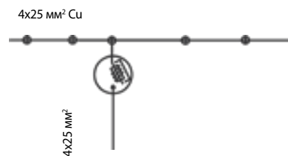
Защита перехода на линию с неизолированными проводниками либо кабельную линию
