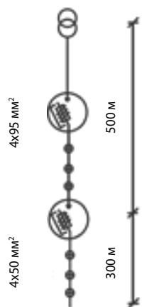
Секционирование участков с разными сечениями
