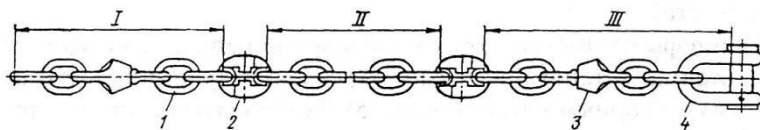
Рис. 9-5. Якорная цепь:
