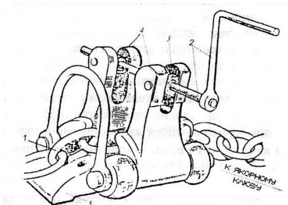
Рис. 9-8. Винтовой стопор:
