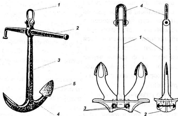
Рис. 9-2. Общий вид адмиралтейского якоря: Рис. 9-3. Устройство якоря Холла:
