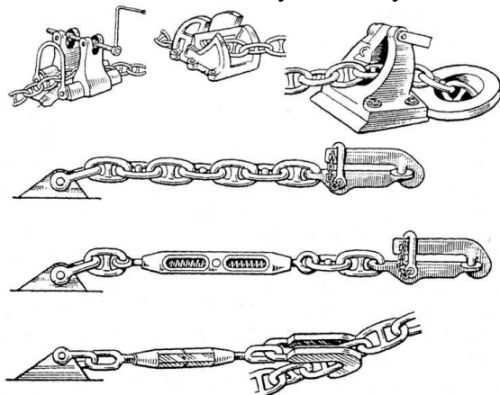
Рис. 9-7. Палубные стопоры.
