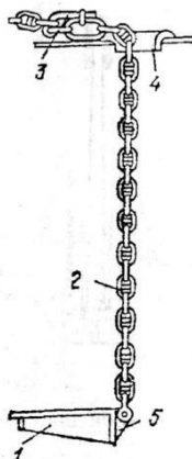
Рис. 9-6. Крепление якорной цепи к корпусу судна с помощью жвака-галса:
