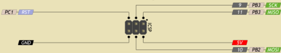
ICSP ATmega16U2
