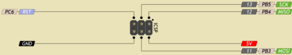
ICSP ATmega328P
