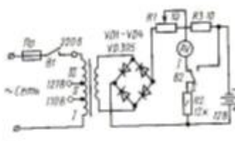
Рисунок 2 Выпрямитель
