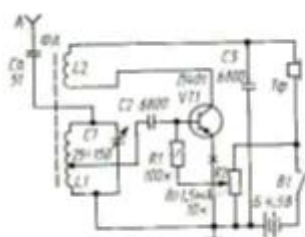
Рисунок 1 Регенеративный графика
