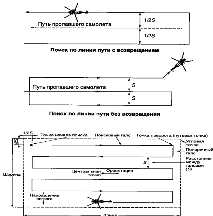
Рис. 8.8. Поиск зигзагом
