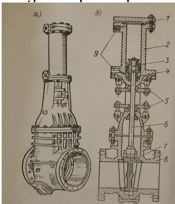
Рис. 21. Клинкет с гидравлическим сервомотором: а — общий вид; б — продольный разрез.
