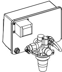
Abb. C-3: Steuerkopf Anschlussnennweite DN 25 (1")
