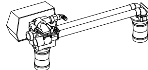
Abb. C-2: Steuerkopf Anschlussnennweite DN 40
